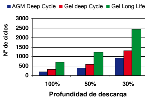
Fig. 2: Duración de vida en ciclos
