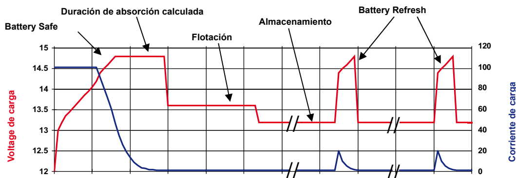
Fig. 4: Carga adaptable en 4 etapas de Victron
